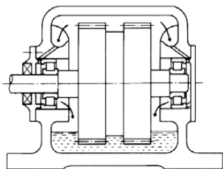
Смазывание разбрызгиванием: коробки передач/редукторы
