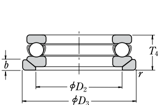
Со сферическим подкладным кольцом
