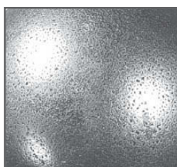
Точечная коррозия
