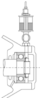
Смазка каплевой подачей: для высоких скоростей
