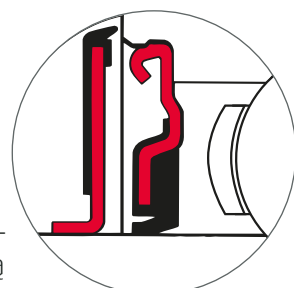
Uszczelka jednowargowa + odrzutnikowa
