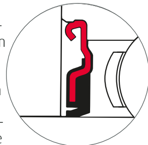
Uszczelka jednowargowa (standardowa)
