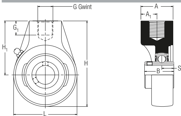
SCHB (gwint BSP) SCH (gwint metryczny)
