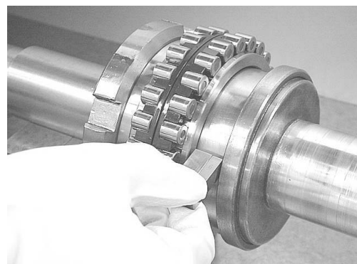
Рис. 1.15 Измерение ширины дистанционного кольца
