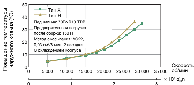
Температурные данные при смазывании воздушно-масляной смазкой
